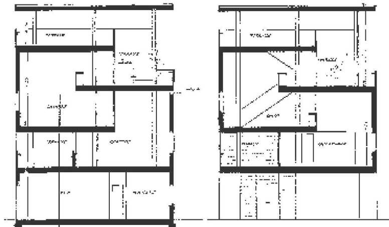
Le Corbusier, Villa Mairea à Carthage (1928, Projekt): Querschnitte. Von Bruno Reichlin als Beispiel einer «solution élégante» ausführlicher vorgestellt. Zwei räumlich wie konstruktiv verschiedene architektonische Konzepte – Maison Citrohan und Maison Dom-ino – werden einander direkt überlagert. Obwohl jedes erkennbar bleibt, sind sie untrennbar; ihre Synthese schafft ein neuartiges Raumgefüge mit modellbildendem Potential.
